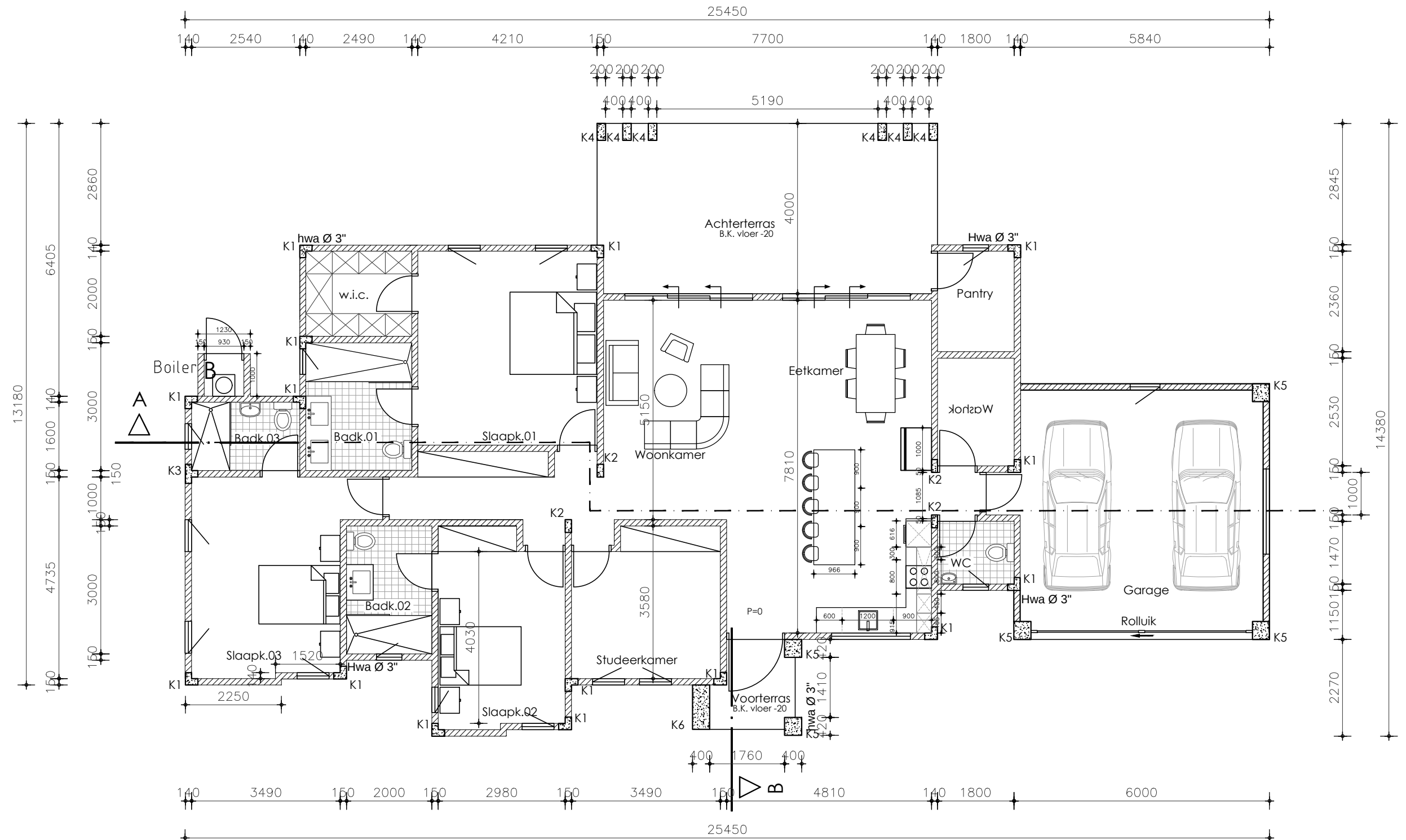
PLATTEGROND WONING-B S C H A A L 1 : 1 0 0 O P P . = 2 4 7 M 2
