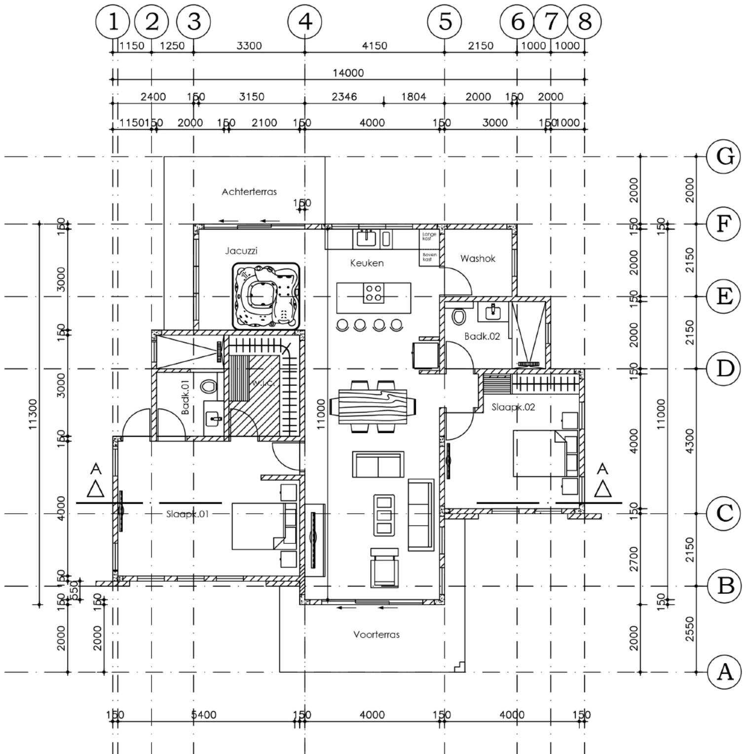
Plattegrond
