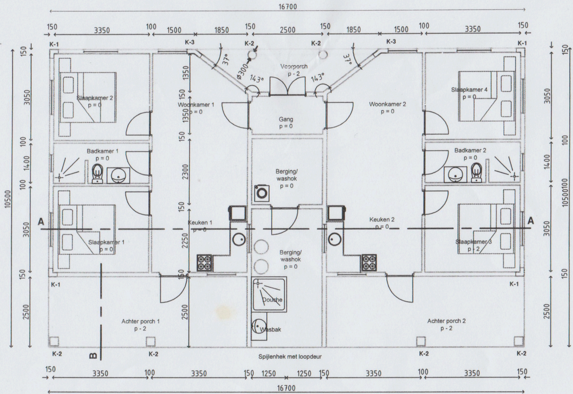
Plattegrond 175,35 m 2 Schaal 1:100
